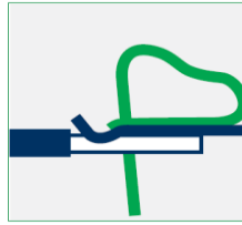
Zugfeder-Anschluss-System ZRK Zugfeder-Prinzip
